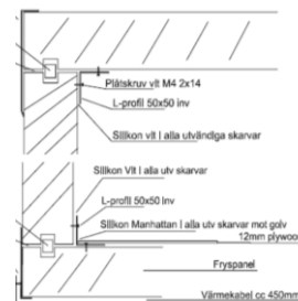
Sektion Tak-vägg-Golv
